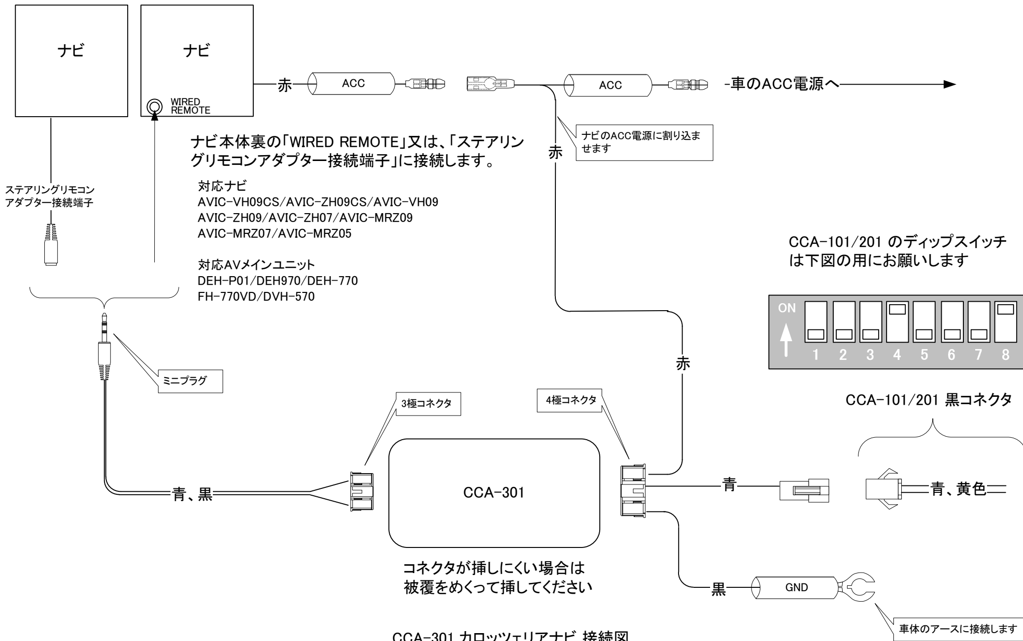
CCA-301 カロツツェリアナビ 接続図
