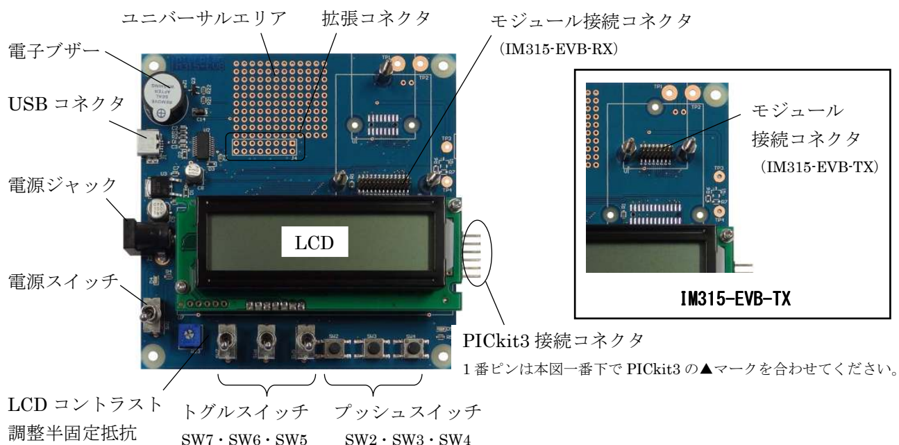
図 1 各部の名称
