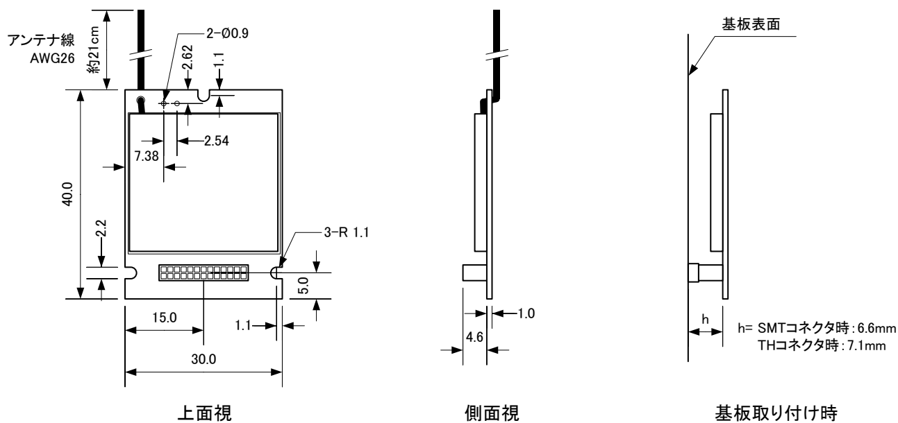
図 1 2 外形寸法図
