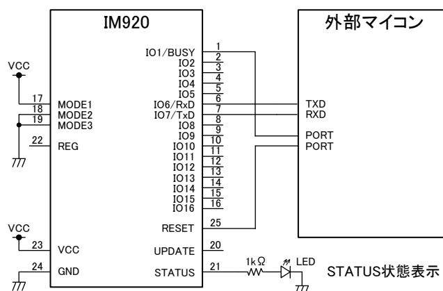
図 12 送受信：データモードの接続例
