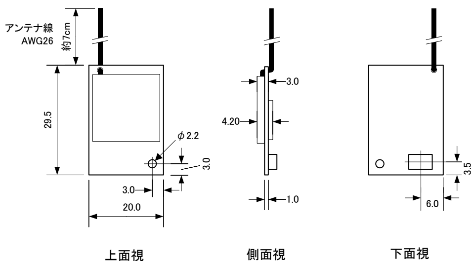
図8 外形寸法図
