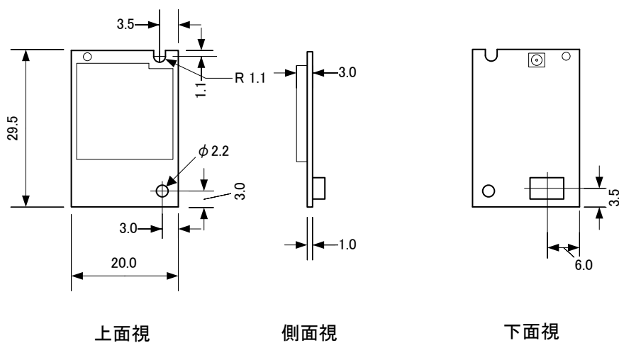
図 11 外形寸法図 (外部アンテナ)
