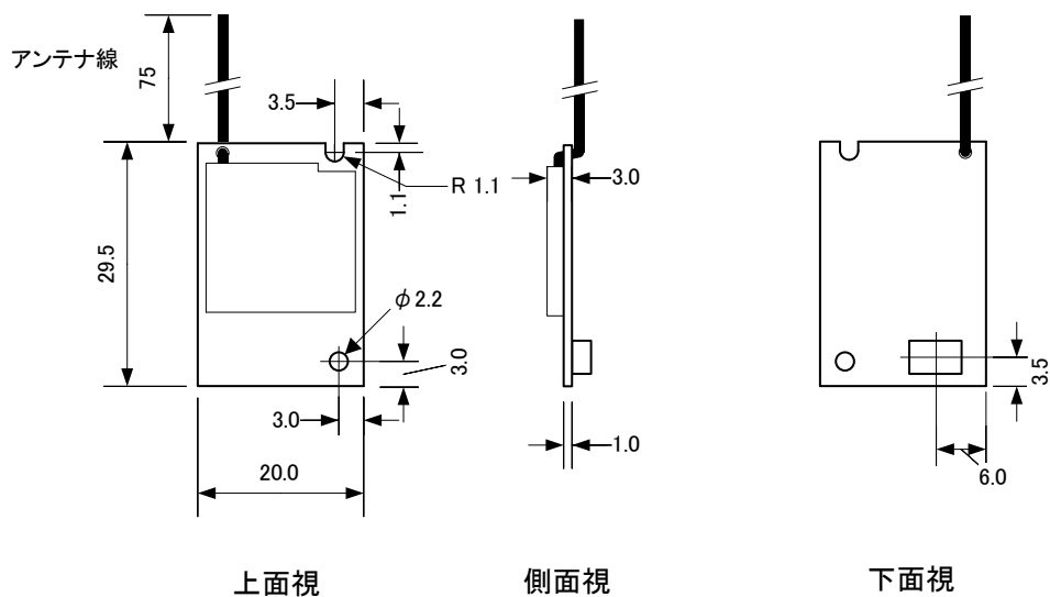
図 10 外形寸法図 (ワイヤーアンテナ)
