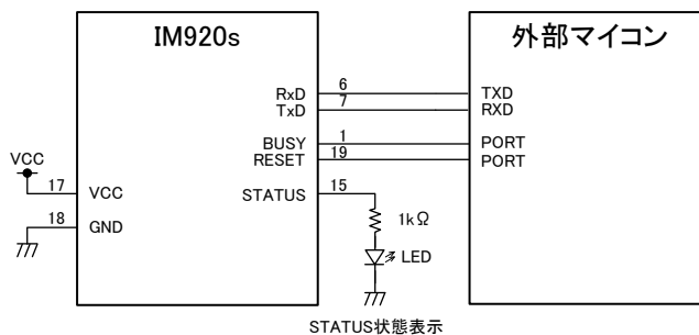
図8 マイコンとの接続例
