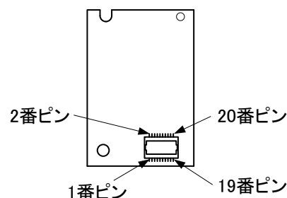
図9 IM920s 端子配置図 (コネクタ面視)
